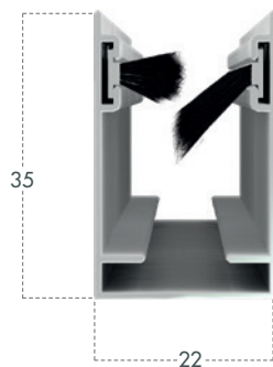
Section coulisse supérieure
