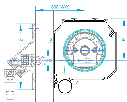
Treuil sortie déportée
