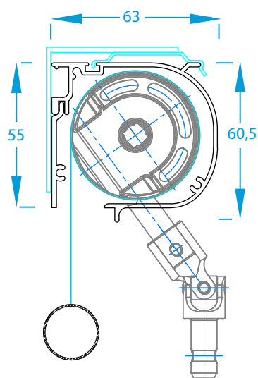
Treuil sortie basse 90°
