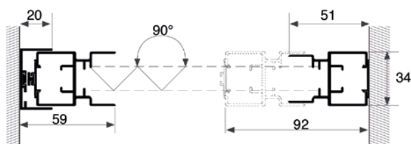
Section Horizontale
