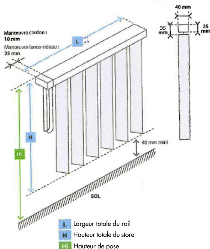
Largeur Rail
