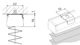
Pose plafond
