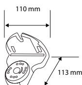
Pose de plafond
