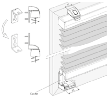
Option pose de face avec plus-value
