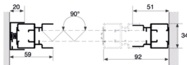
Section Horizontale
