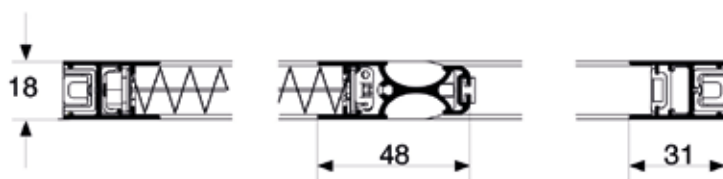
Section Horizontale
