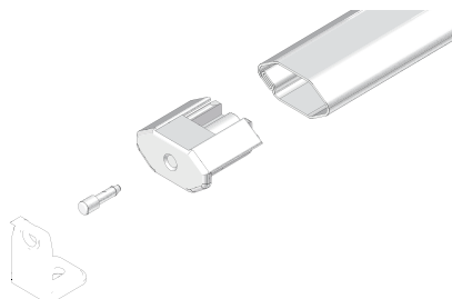
Bloquent barre finale pour ouvrant et double vitrage obligatoire pour largeur de 300 mm et moins.
